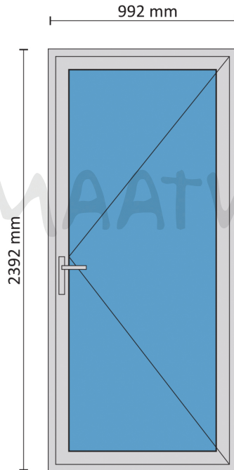
Buitenaanzicht
