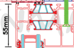
Aansluitdetail nr. K10
