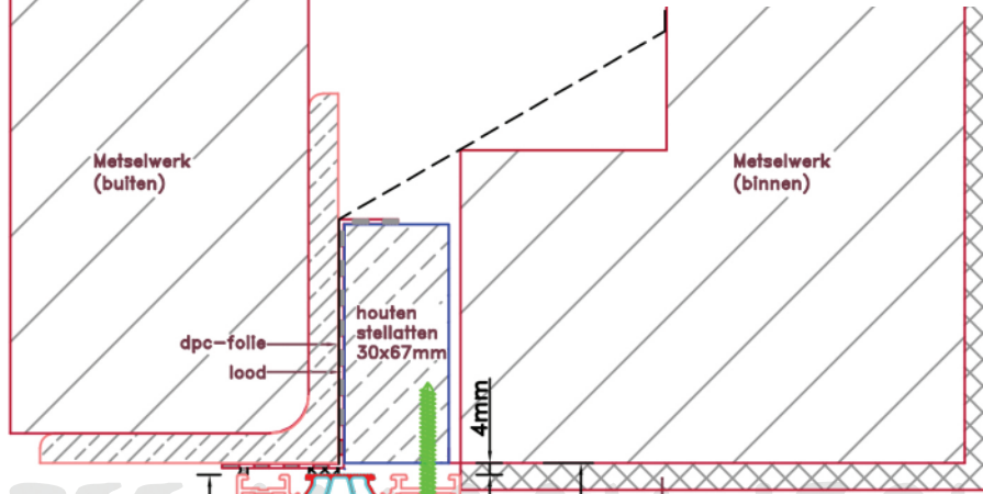
Aansluitdetail nr. K10
