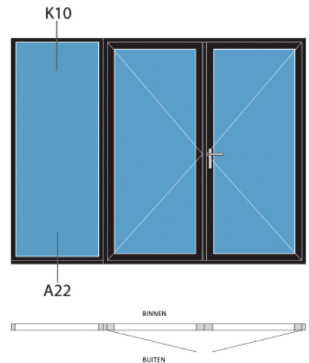
Doorsnedes dubbele deur STD420
