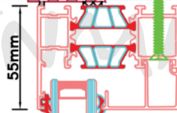
Aansluitdetail nr. K10
