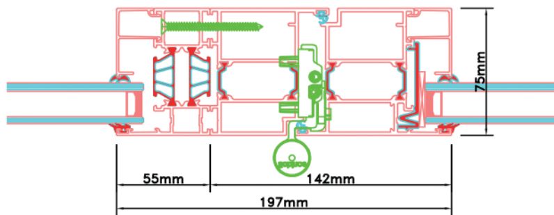
Aansluitdetail nr. A18
