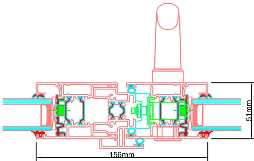
Aansluitdetail nr. S74
