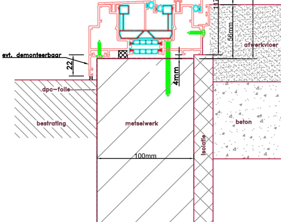
Aansluitdetail nr. S45 Verzonken dorpel
