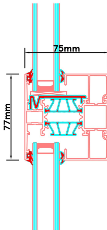
Aansluitdetail nr. K15
