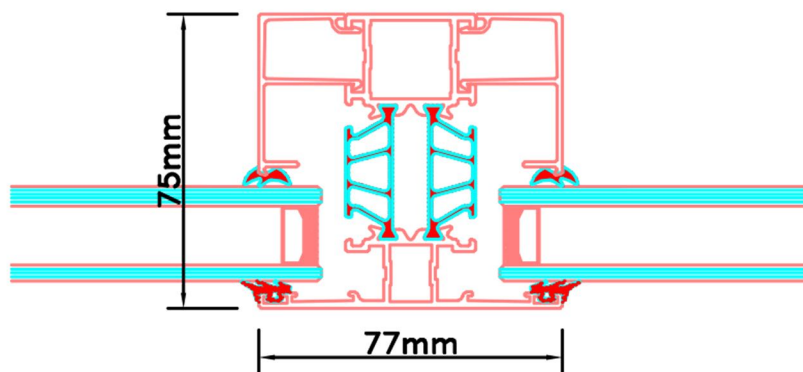
Aansluitdetail nr. K14
