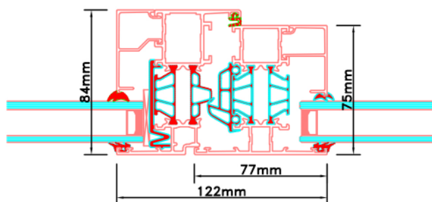
Aansluitdetail nr. D18
