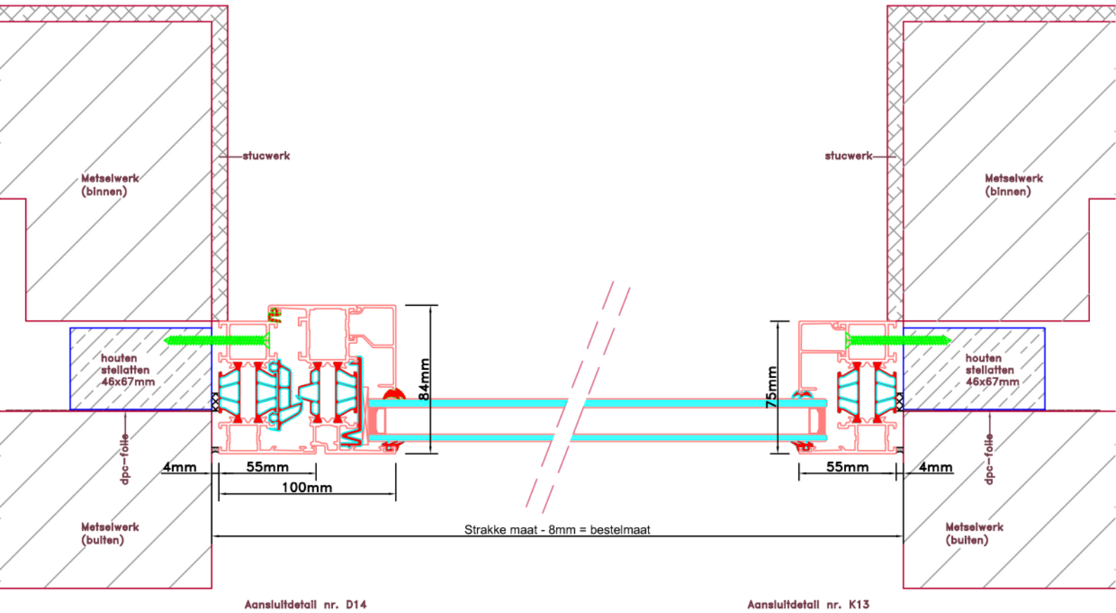
Aansluitdetail nr. D14
