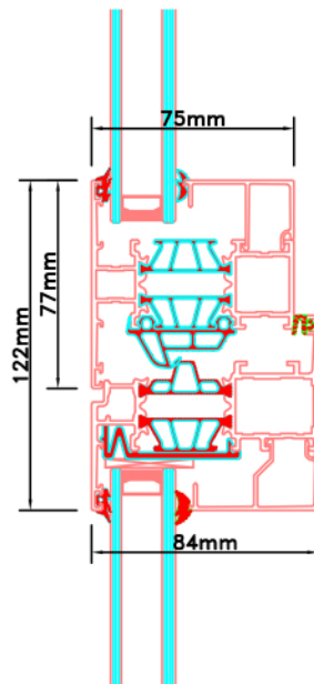
Aansluitdetail nr. D22
