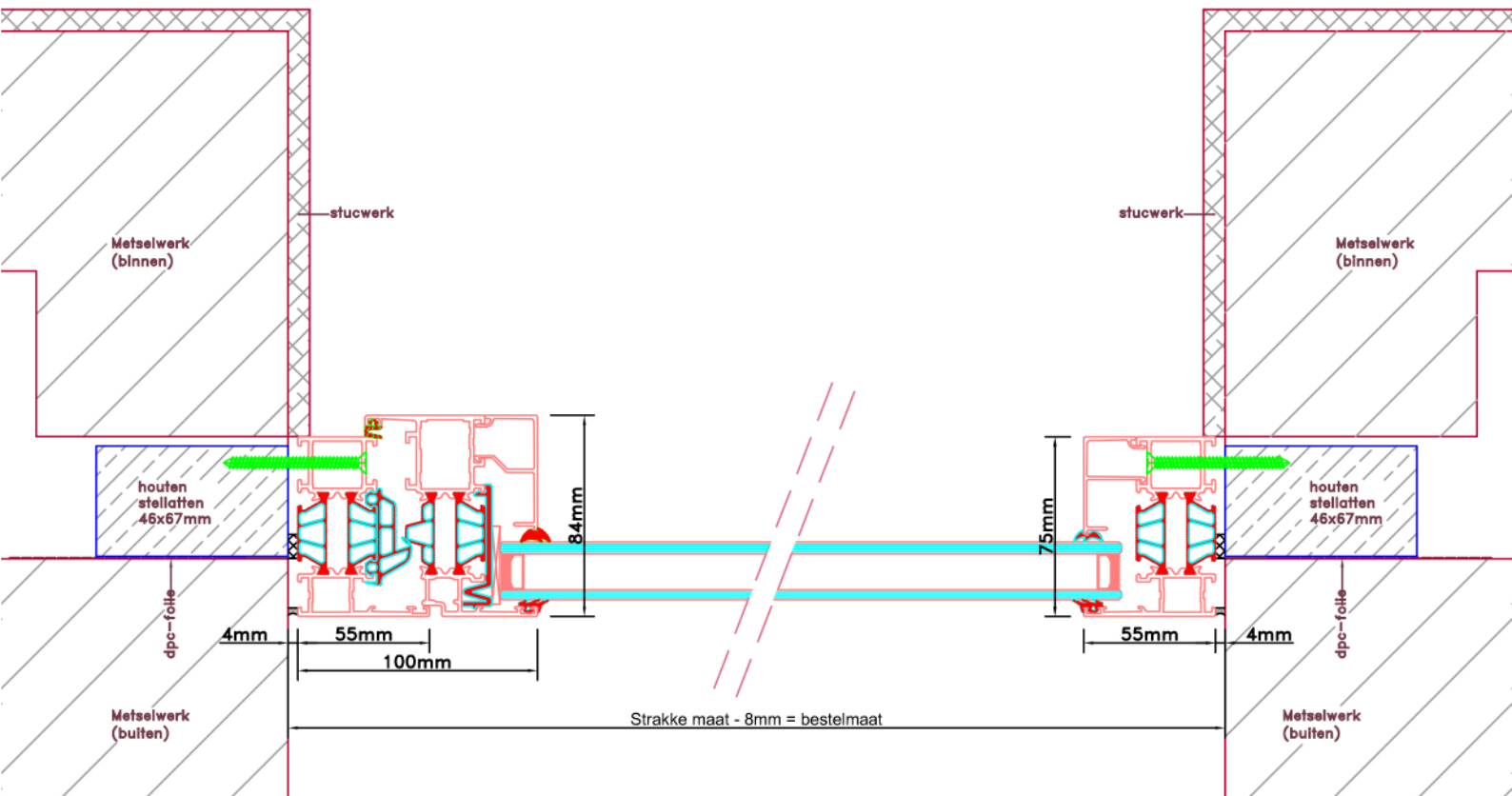
Aansluitdetail nr. D14
