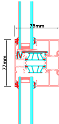
Aansluitdetail nr. K15
