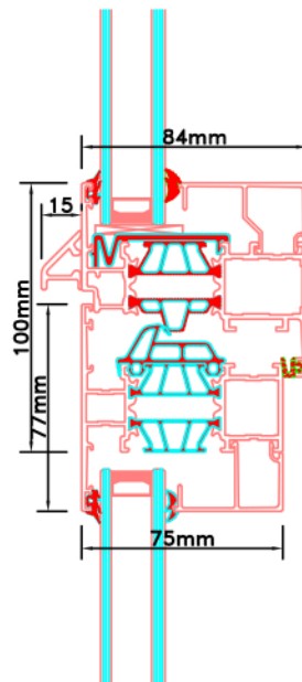
Aansluitdetail nr. D23
