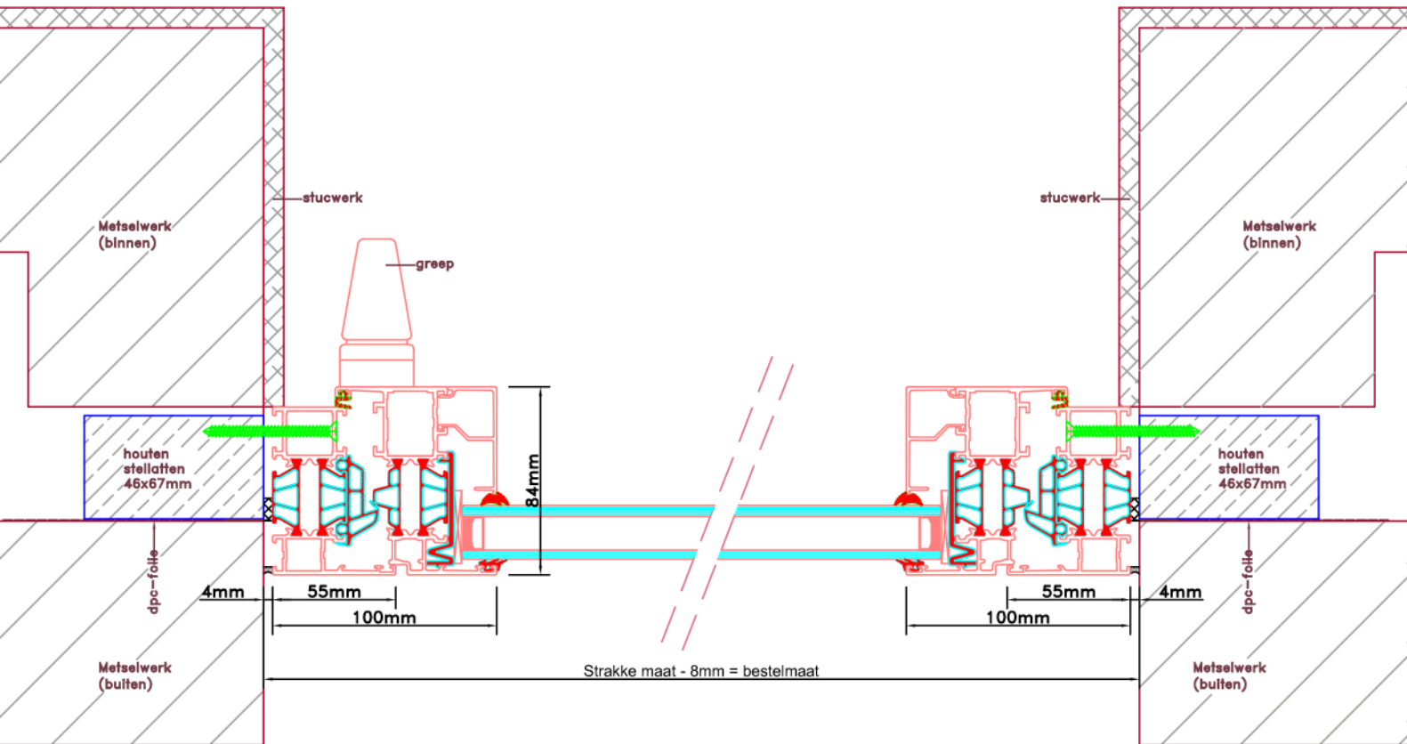
Aansluitdetail nr. D12
