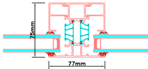
Aansluitdetail nr. K14
