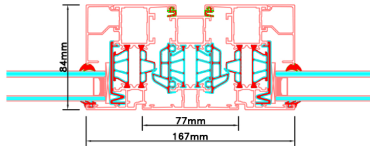
Aansluitdetail nr. V14
