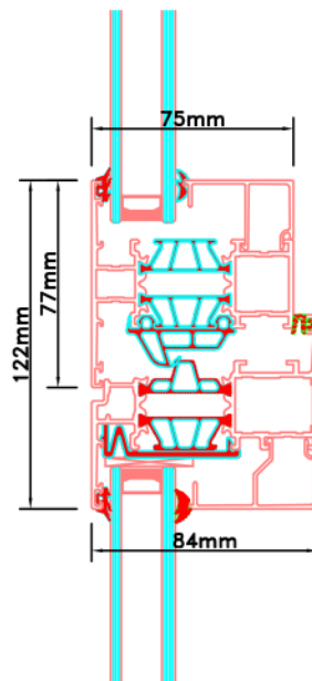
Aansluitdetail nr. D22
