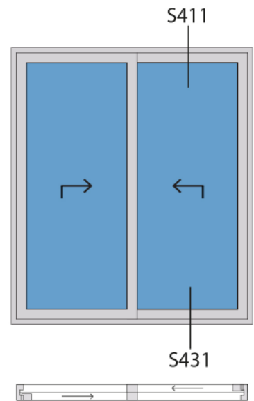
Doorsnedes hefschuifpui S227
