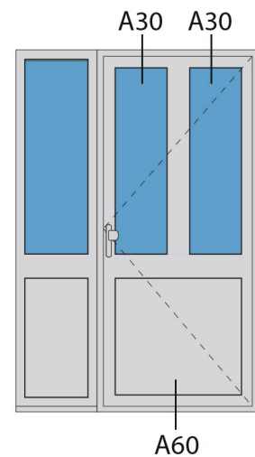
Doorsnedes voordeur V196 binnendraaiend
