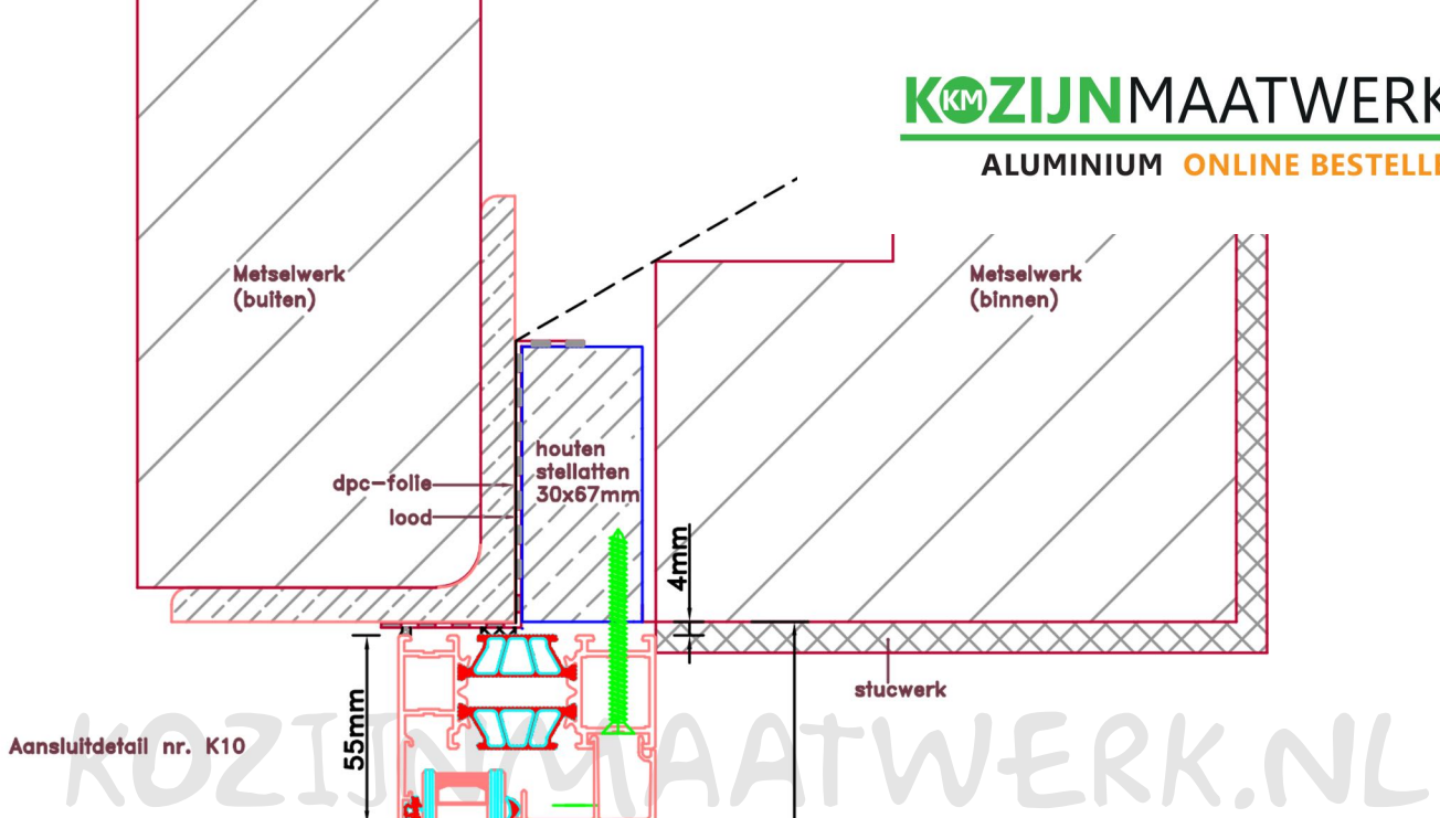
Doorsnedes voordeur V194 binnendraaiend
