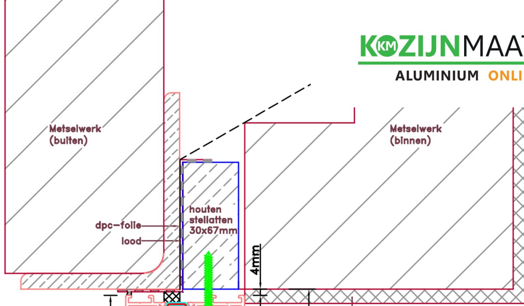
Aansluitdetail nr. A10
